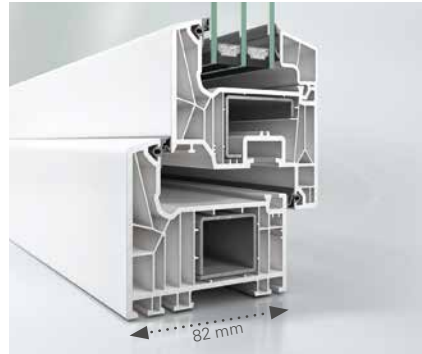
Hohe Basissicherheit: Die erhöhte Bautiefe und weit innen liegende Beschläge entziehen die Verschlusselemente dem Angriff der Einbrecher.
